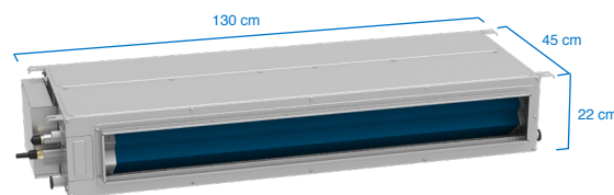
Unidad Monofásica 24 Kbtu
