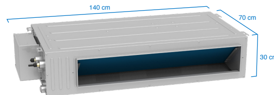
Unidades Trifásicas 48 y 60 Kbtu
